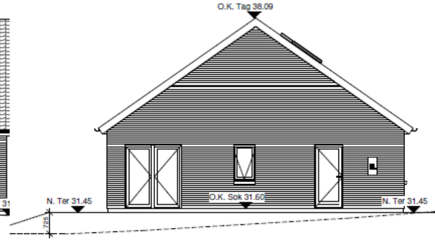
Facade mod Øst
